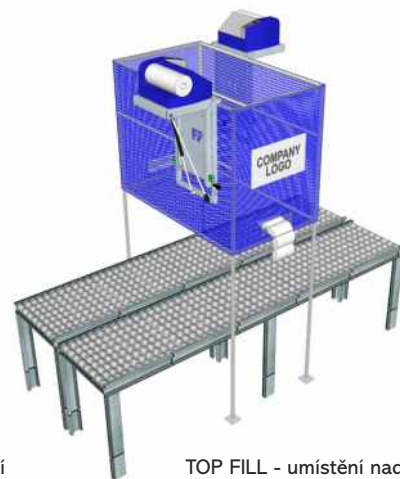
TOP FILL - umístění nad balícím stolem
